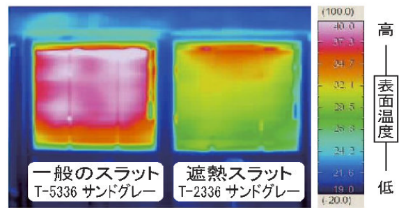
ブラインド表面の温度差 (サーモカメラで撮影)
